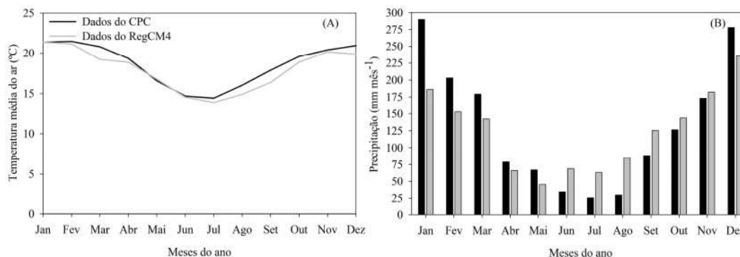
Figura 3: Ciclo anual de temperatura média do ar (A) e precipitação acumulada mensal (B) provenientes dos dados do Climate Prediction Center (CPC) e simulados pelo modelo regional de previsão climática RegCM4 para o período de 1979-2005 para Itajubá (MG). Em cinza, dados do modelo RegCM4, em preto, dados do CPC.
