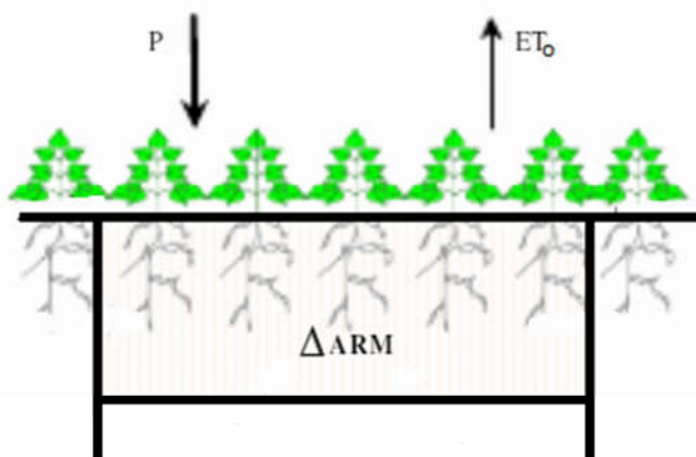
Figura 2: Representação do balanço hídrico climatológico simplificado.
