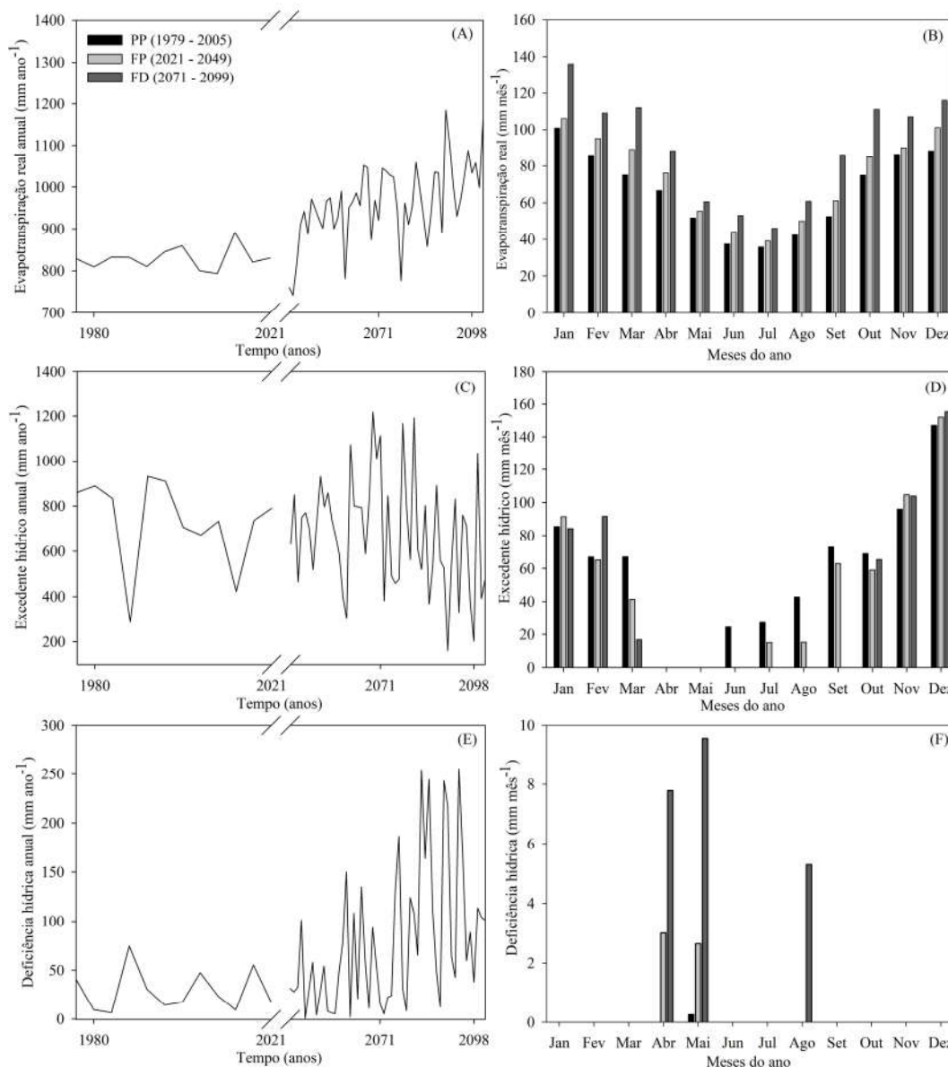
Figura 5: Variação temporal simulada (1979-2005) e projetada (2021 – 2099) para a evapotranspiração real anual (A), excedente hídrico anual (C) e deficiência hídrica anual (E) para o cenário forçante RCP 8.5; e padrão mensal da evapotranspiração real acumulada (B), excedente hídrico (D) e deficiência hídrica (F) para Itajubá (MG), considerando o período atual (1979 – 2005), futuro próximo (2021-2049) e futuro distante (2071-2099) para o cenário forçante 8.5. Devido aos valores, os eixos das variáveis estão em escalas diferentes.
