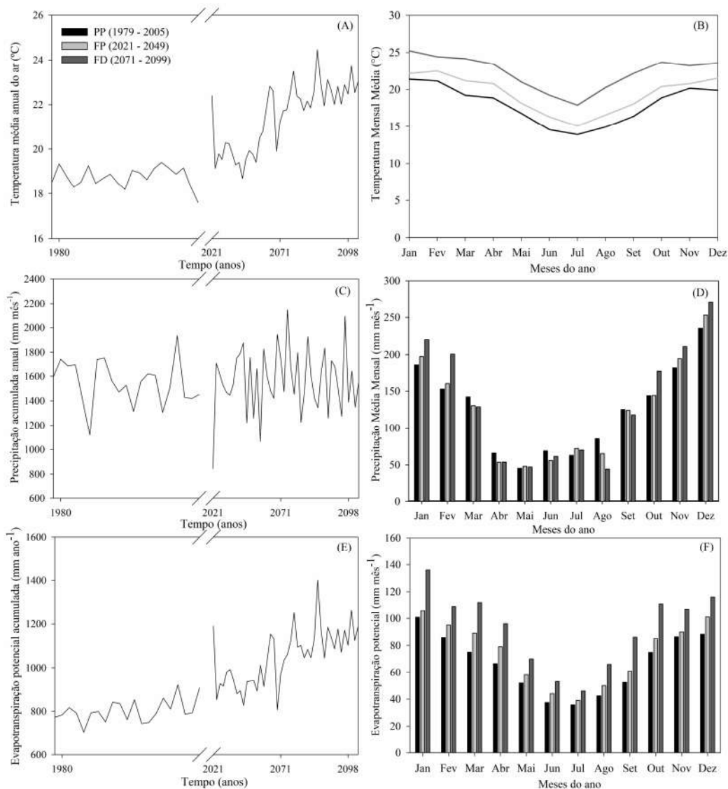
Figura 4: Variação temporal simulada (1979-2005) e projetada (2021 – 2099) e padrão mensal da temperatura média do ar (A,B), precipitação acumulada anual/mensal (C,D), evapotranspiração acumulada anual/mensal (E,F) para Itajubá considerando o período atual (1979 – 2005), futuro próximo (2021-2049) e futuro distante (2071-2099) obtidas pelo modelo regional RegCM4 e cenário forçante 8.5. Devido aos valores, os eixos das variáveis estão em escalas diferentes.
