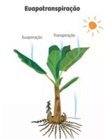
Figura 1: Representação da evapotranspiração.
